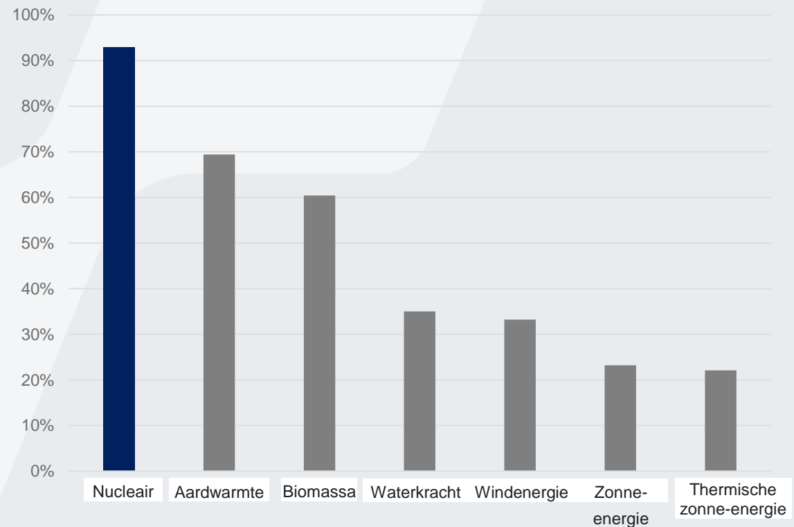
Capaciteitsfactor van koolstofarme energie, %
