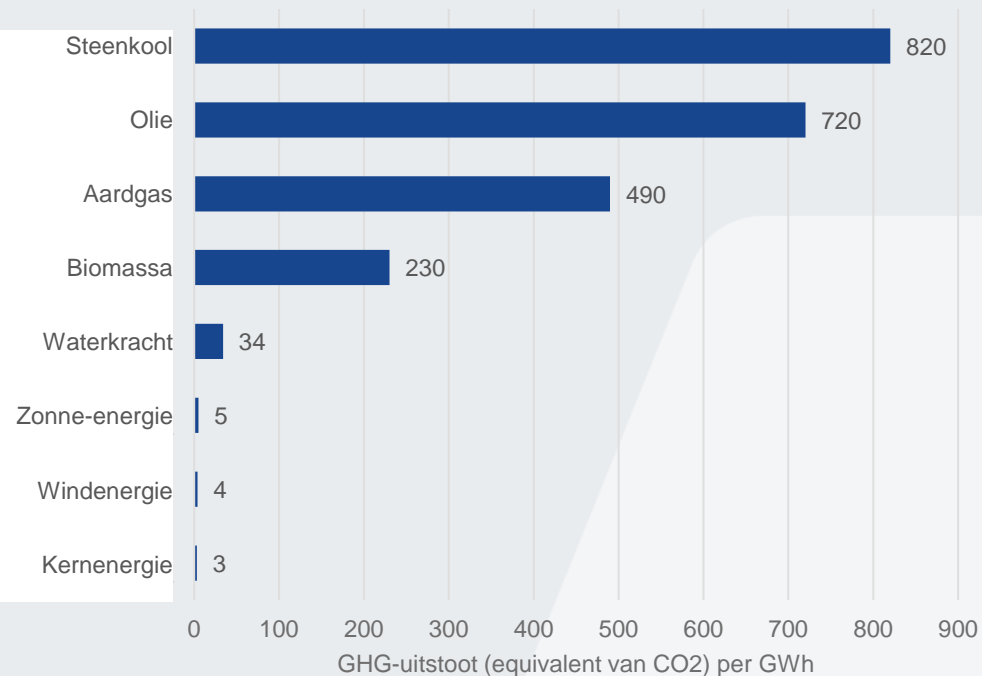
CO 2 -voetafdruk gedurende de levenscyclus van een elektriciteitscentrale.
